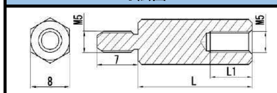
寸法図
