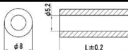
寸法図
