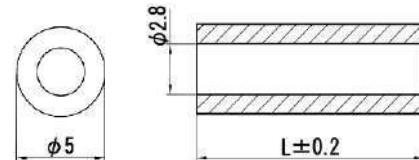
寸法図
