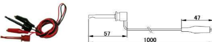
TLA-107 ICクリップL⇔シールドクリップM 【半田付け】
