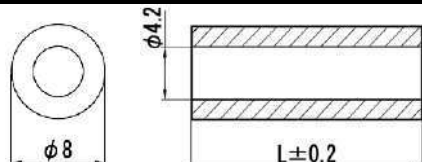
寸法図
