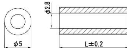
寸法図
