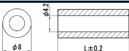
寸法図
