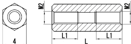
寸法図
