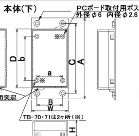
本体(下)
