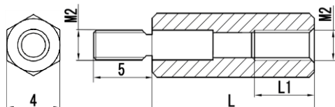
寸法図
