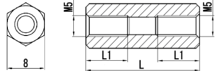
寸法図
