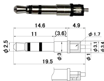
φ2.5-3極(ステレオ)プラグ
