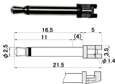
φ2.5-2極(モノラル)プラグ
